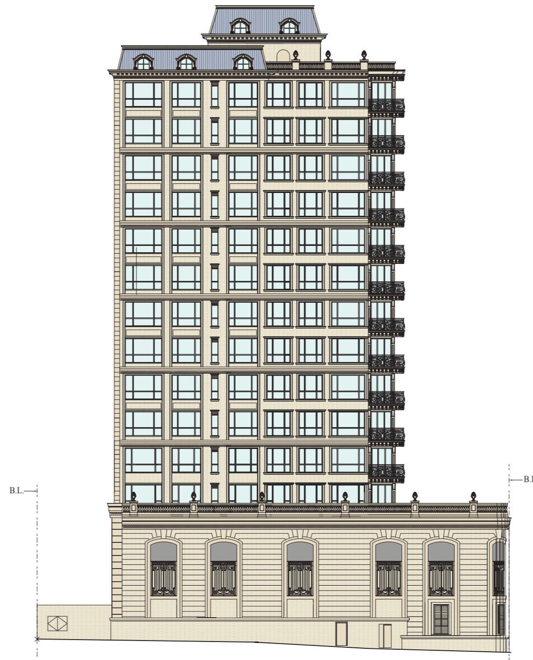
東南面立面圖 SOUTH EAST ELEVATION
