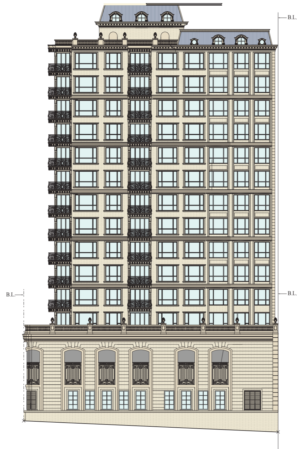
東北面立面圖 NORTH EAST ELEVATION
